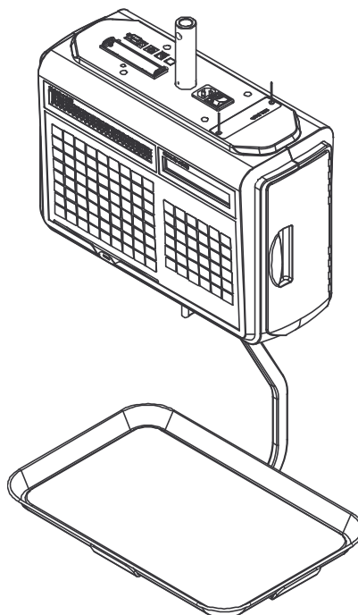
Рисунок 1.4 – Контурный вид подвесной модификации (CL5000J-IH)
