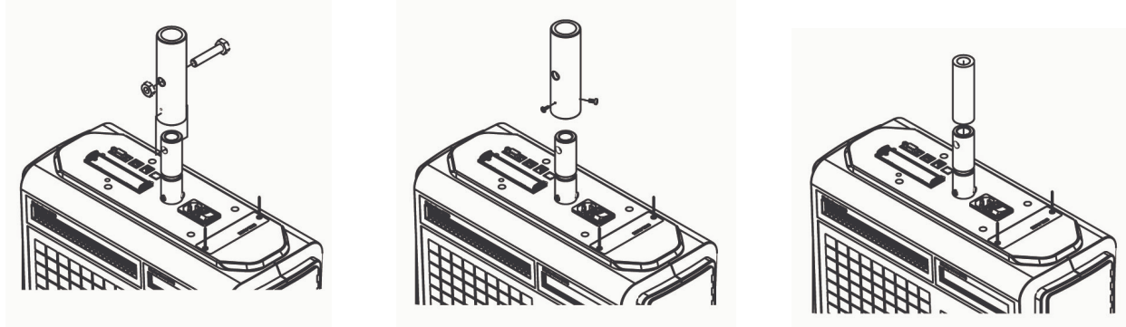
Рисунок 1.11 – Порядок монтажа верхних кронштейнов
